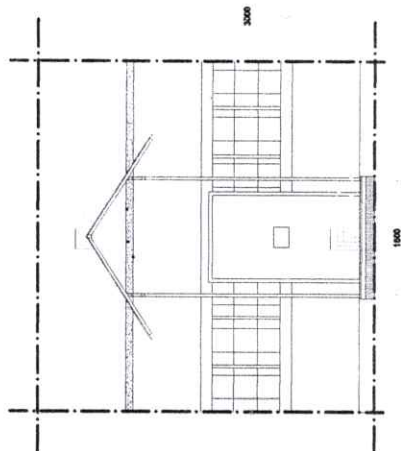
Detail Rencana Canopy Depan Pintu Masuk Pasien SKALA 1:100
